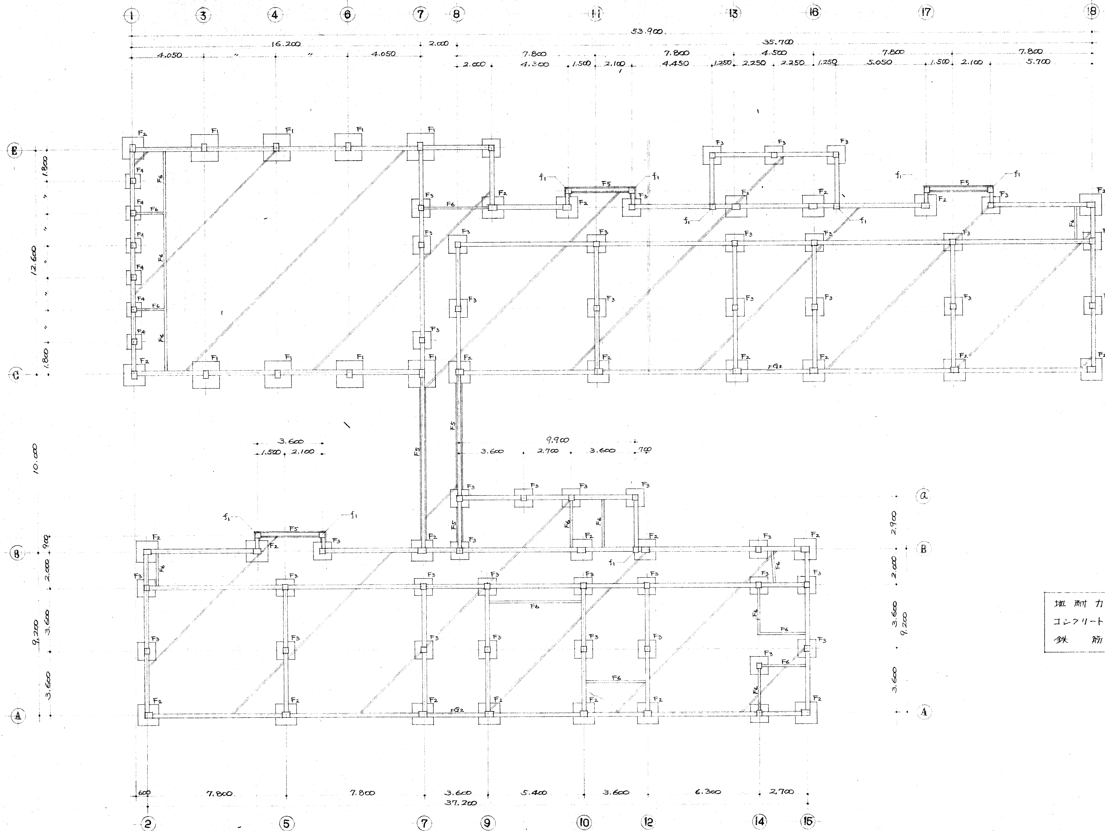
基礎伏図 1/100 (註) 通芯、列芯は全て壁芯とする。特記なき梁中梁は全てF51とする。
