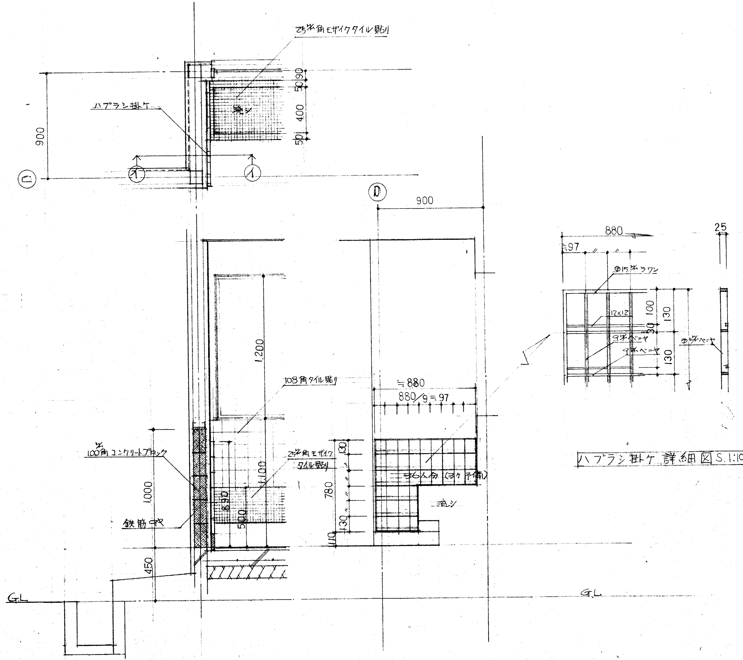
①-① 断面詳細図 6:1:20
