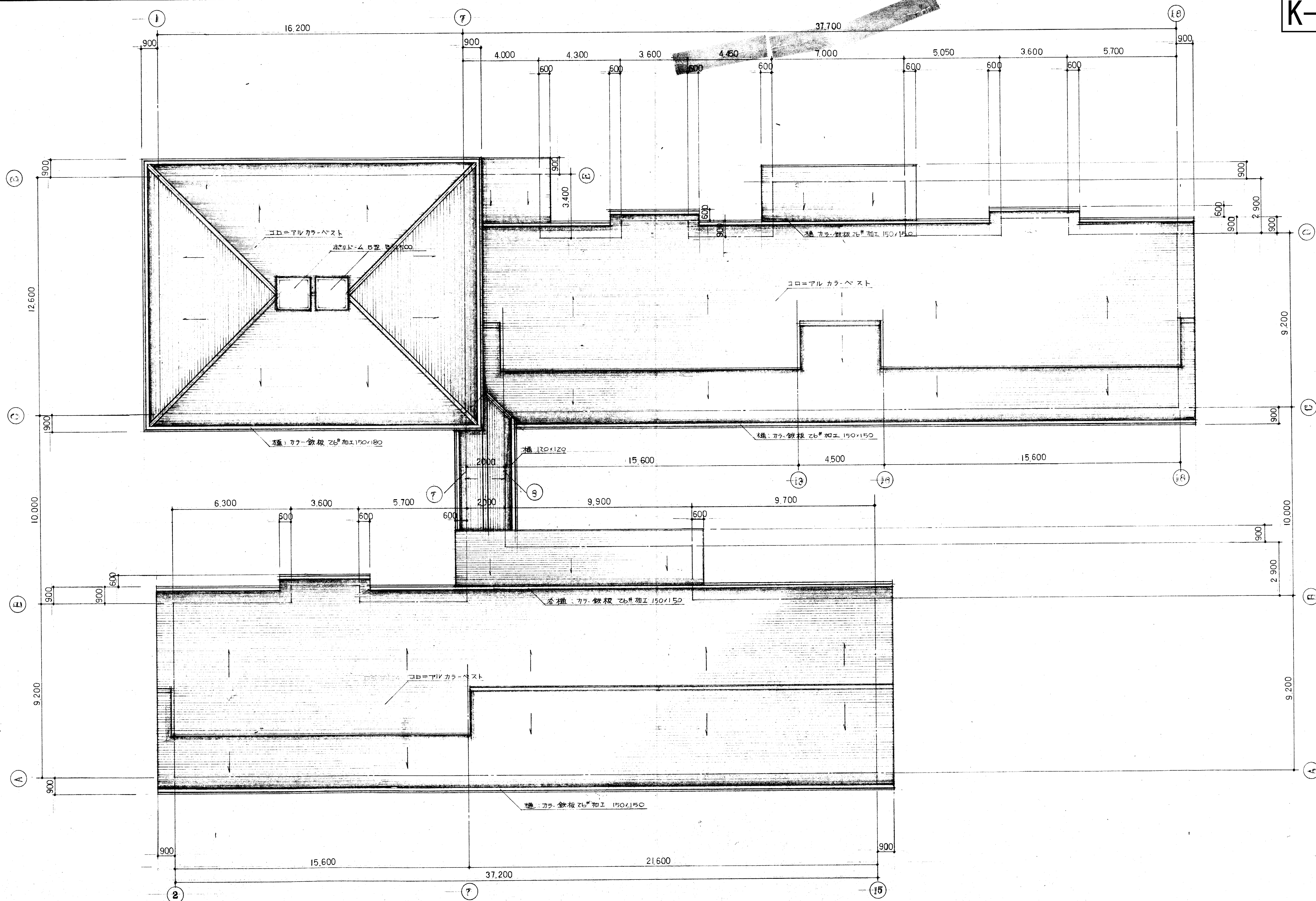
屋根伏図 S:1:100
