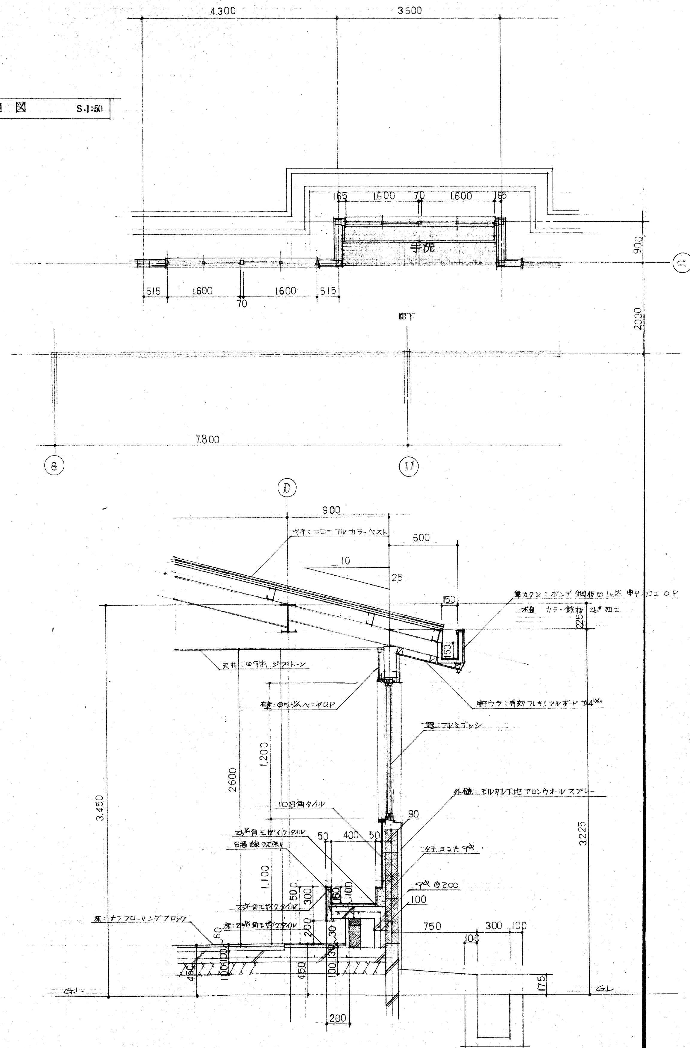
手洗断面詳細図 8.1:20
