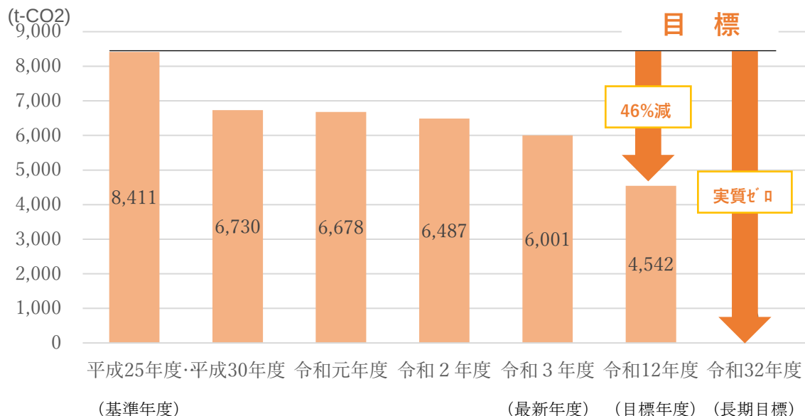
図表4-1-1 温室効果ガス排出量実績と目標
