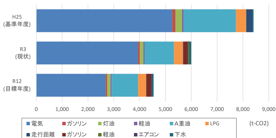
図表4－2－2 目標達成のための活動量と排出量
