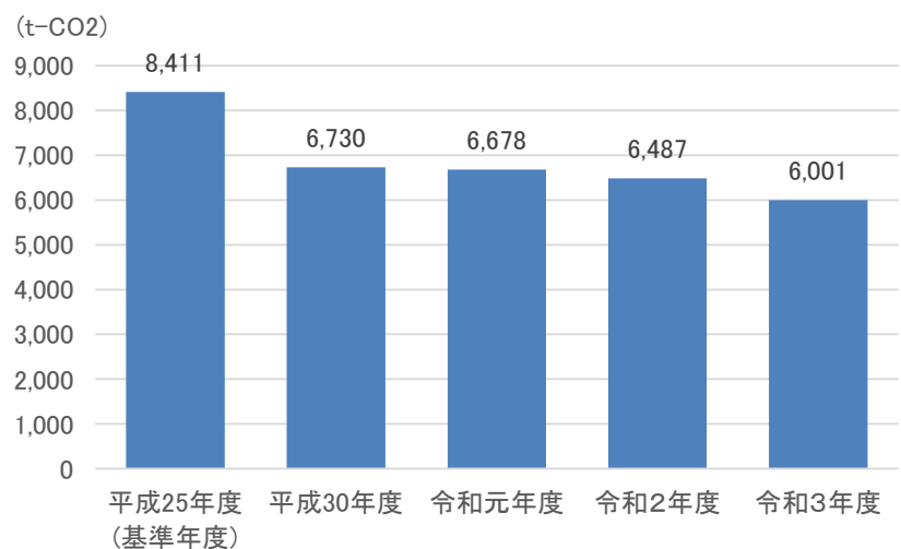
図表2-3-3 温室効果ガス排出量の推移
