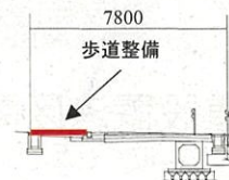
標準断面図
