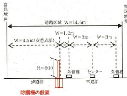
標準横断図
