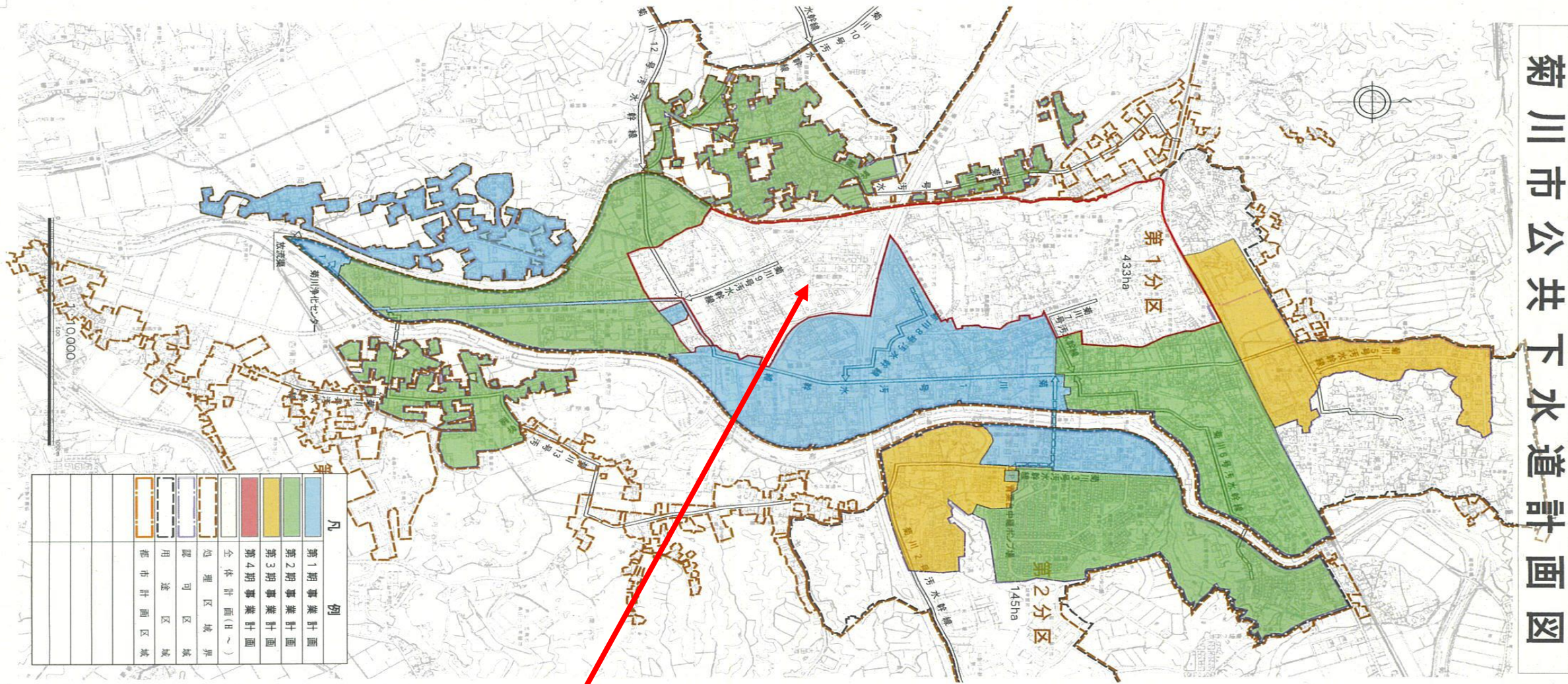
A-07-001 菊川処理区管渠整備
