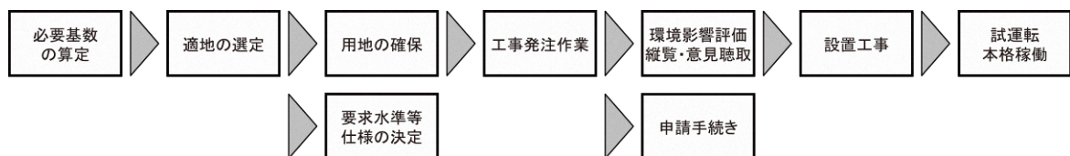
図 4-1-2 仮設焼却炉設置フロー
